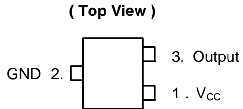
(2) SC59
