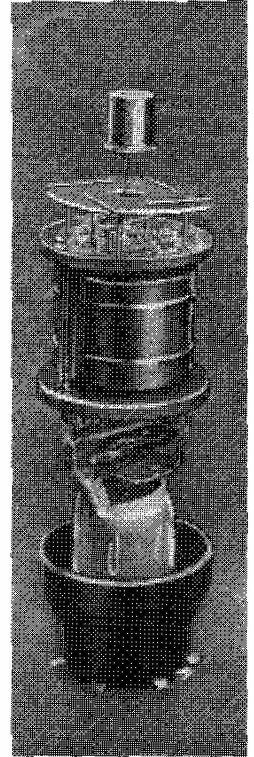
Construction intérieure de l'octode changeuse de fréquence KK 2.
