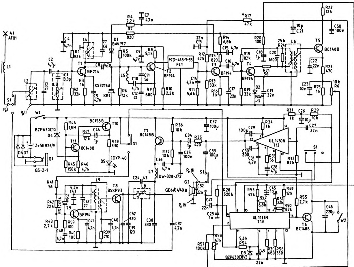
Rys. 10.2. Schemat ideowy radiotelefonu Tukan
