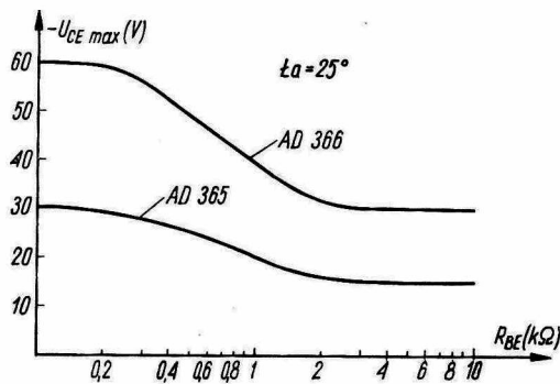
Rys. 3. Zależność maksymalnego napięcia kolektor — emiter od oporności między bazą i emitrem
