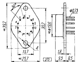
Układ scalony w obudowie typu CE51 (TO-3)
