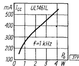
Prąd zasilania w funkcji mocy wyjściowej
