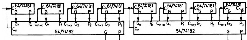
Rys. 3.118. Dwupoziomowa generacja przeniesień w 32-bitowym układzie arytmetycznym
