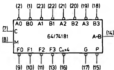
Symbol graficzny układu 64/74181 przy założeniu, że sygnałem aktywnym jest stan niski (L)
