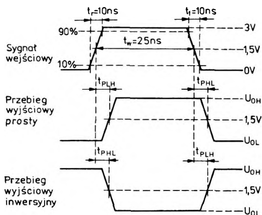
Przebiegi określające pomiary parametrów dynamicznych
