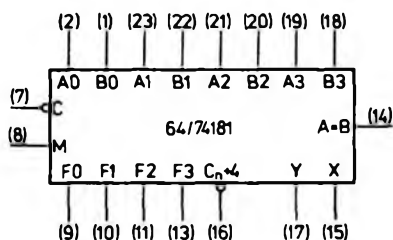
Symbol graficzny układu 64/74181 przy założeniu, że sygnałem aktywnym jest stan wysoki (H)
