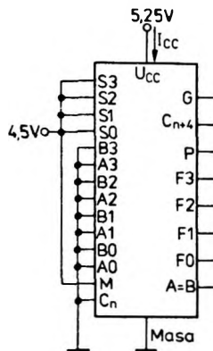
Układ pomiarowy G. Pomiar I_{CC}
