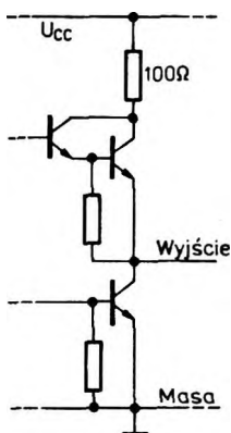
Typowy schemat obwodu każdego wyjścia z wyjątkiem wyjścia A = B
