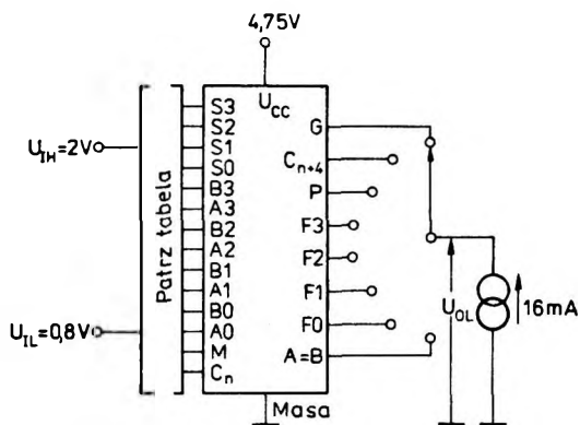
Układ pomiarowy B Pomiary U_{OL}
