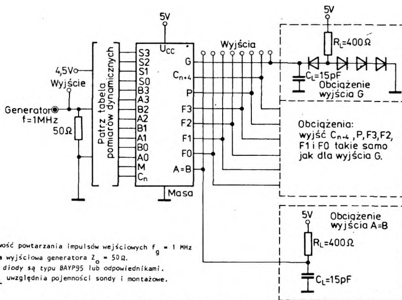
Układ pomiarowy H. Pomiary parametrów dynamicznych
