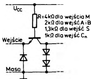
Uproszczony schemat obwodu każdego wejścia
