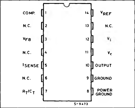
DIP-14 / SO-14.
