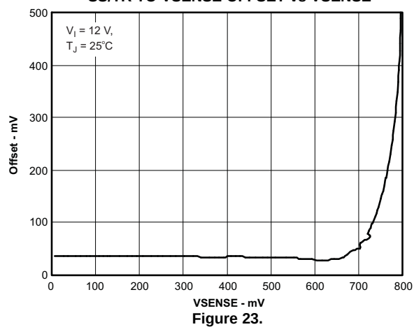
SS/TR TO VSENSE OFFSET vs VSENSE
