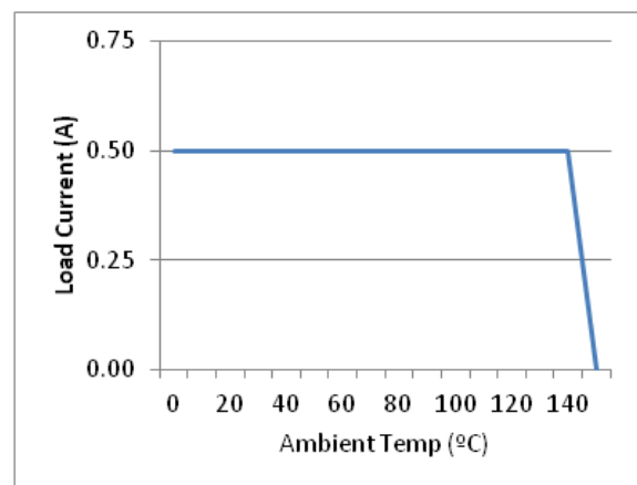
Figure 13. Q1 SOA at VGS_Q1=-1.2V
