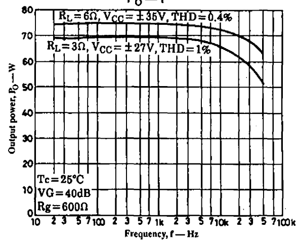
P_o - f
