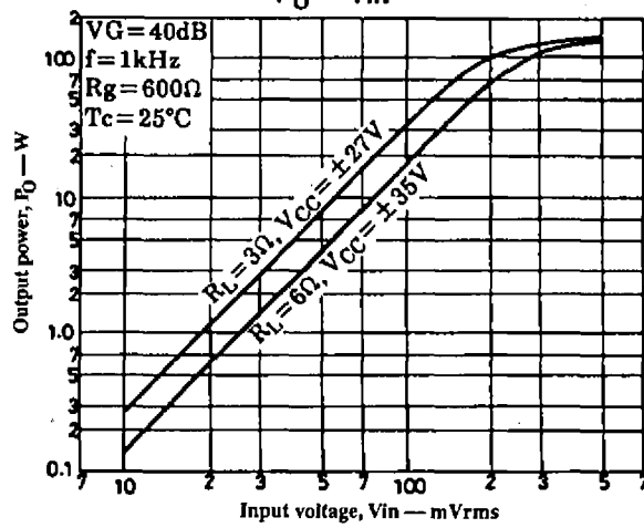
P_o - V_{in}
