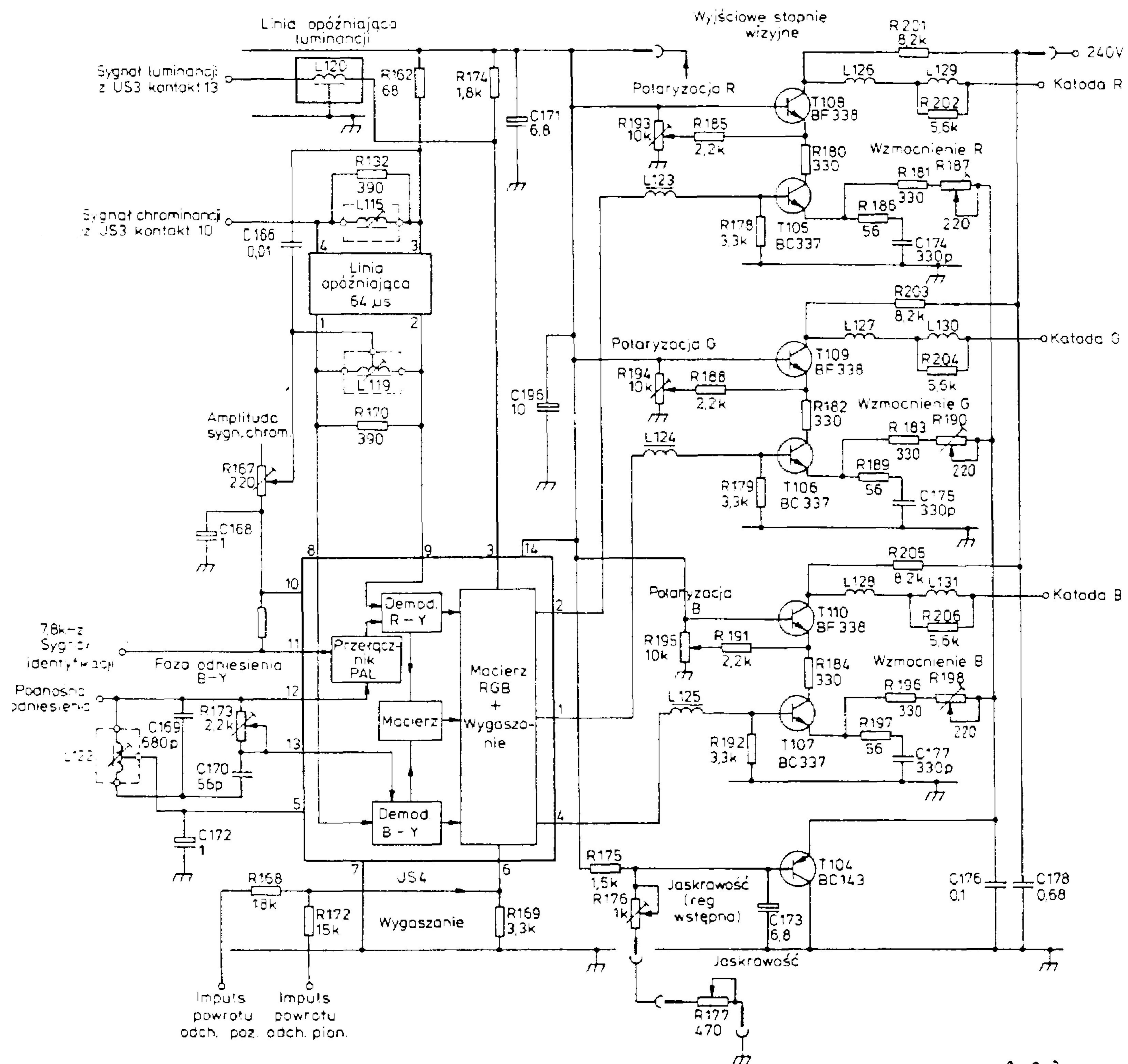
Całkowity układ wyjściowy RGB (chassis 9000 firmy Ferguson)
