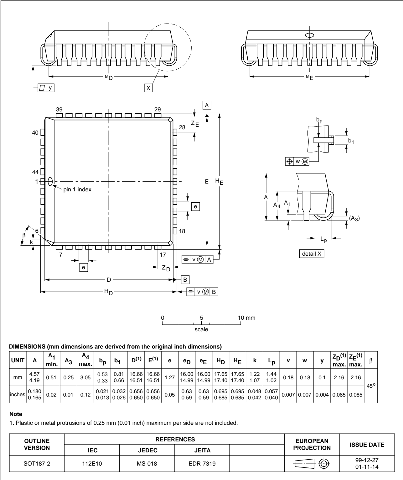
Fig 25. PLCC44 (SOT187-2).
