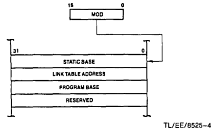
FIGURE 2-4. Module Descriptor Format
