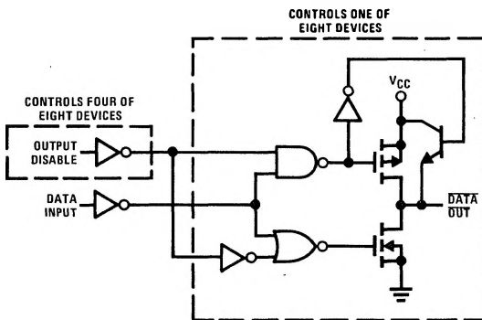
MM54C240/MM74C240
