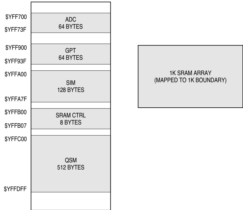
Z1 ADDRESS MAP
