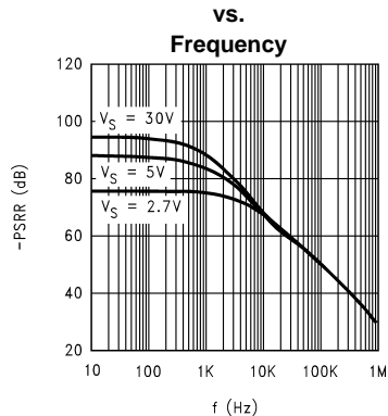
-PSRR
