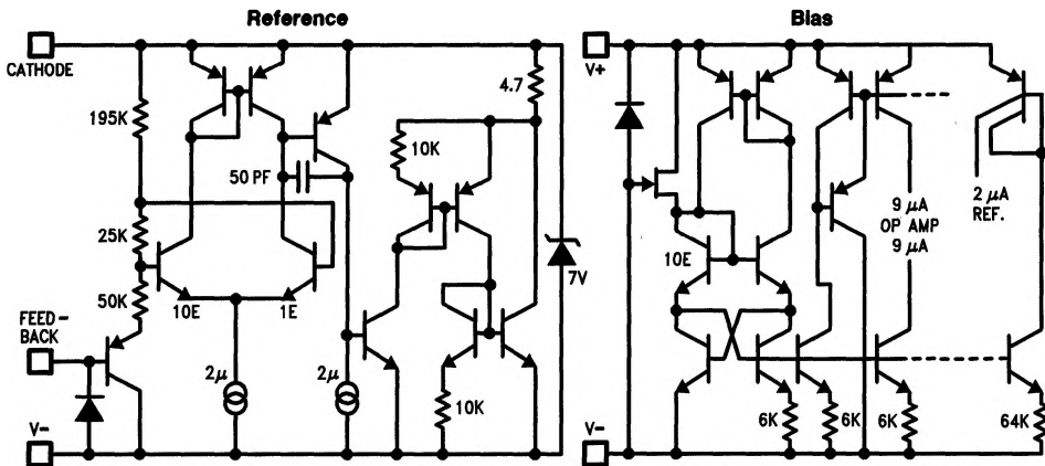
TL/H/9226-4
