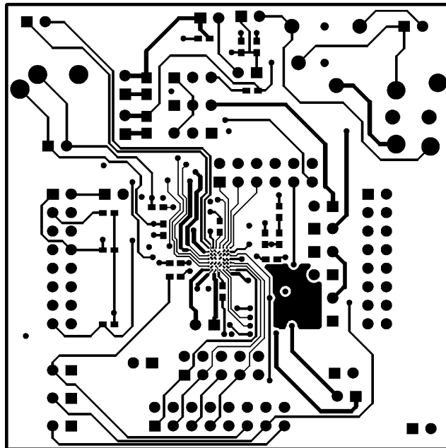
Figure 29. Top Layer
