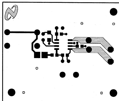
Figure 25. Top Layer
