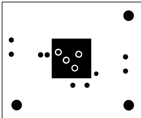
Figure 22. Inner Layer V DD
