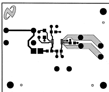
Figure 28. Top Layer
