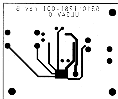
Figure 26. Bottom Layer
