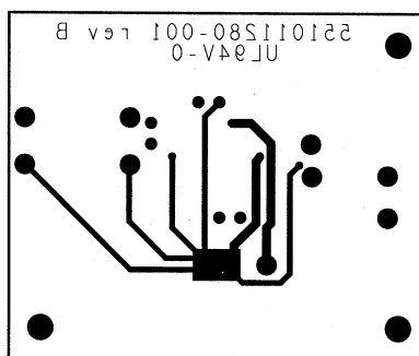
Figure 29. Bottom Layer
