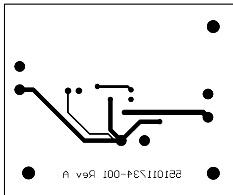
Figure 20. Bottom Layer
