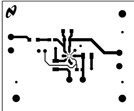
Figure 19. Top Layer
