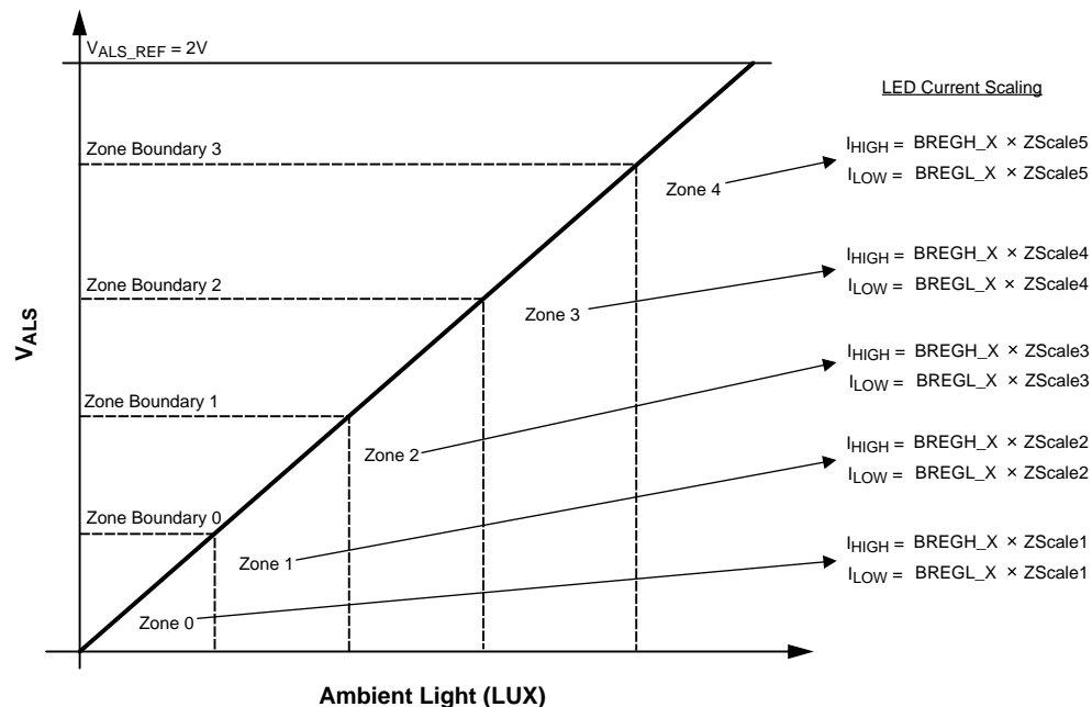
Figure 16. ALS Controlled Pattern Current Scaling
