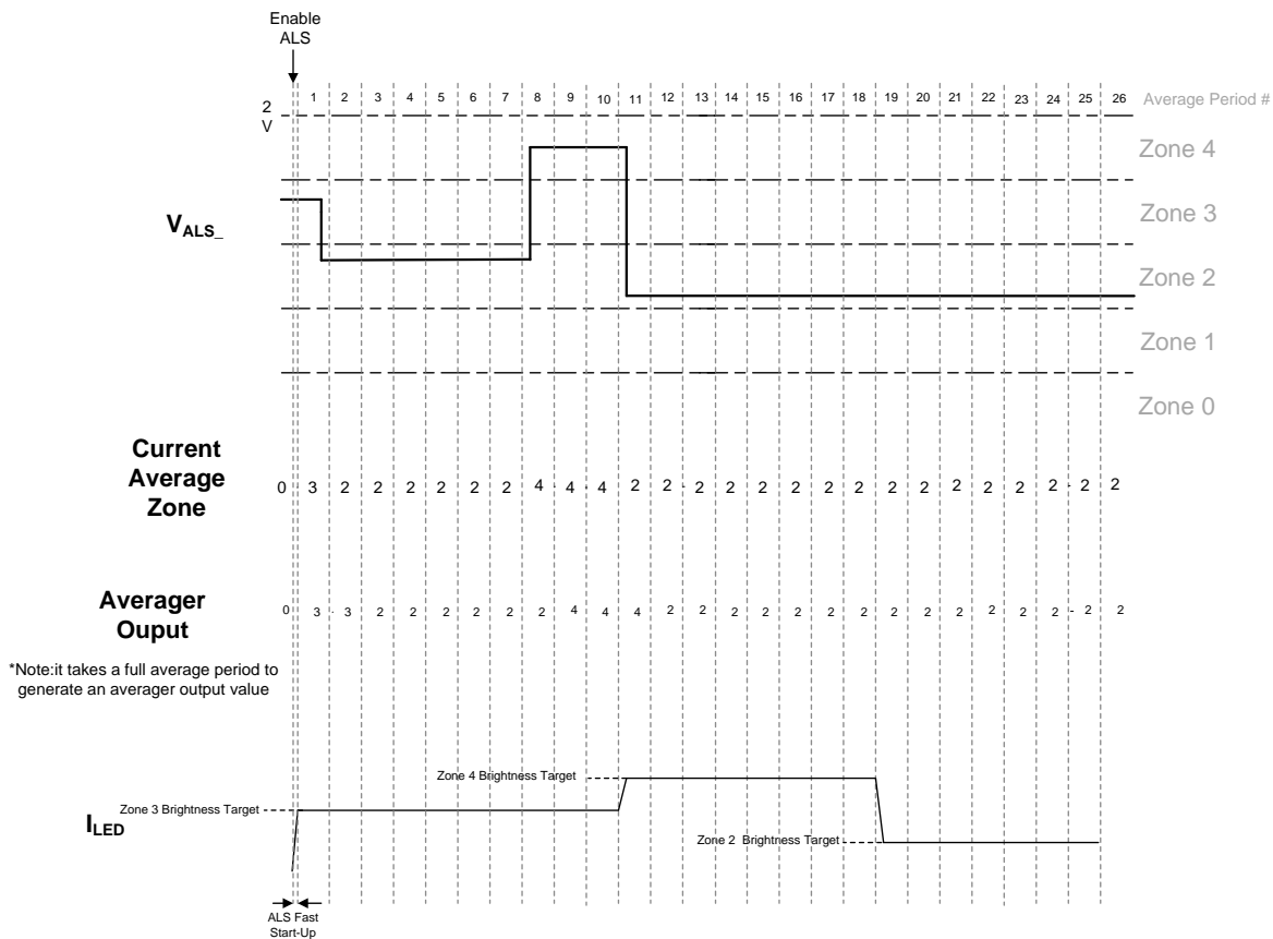
Figure 14. ALS Down-Delay Control
