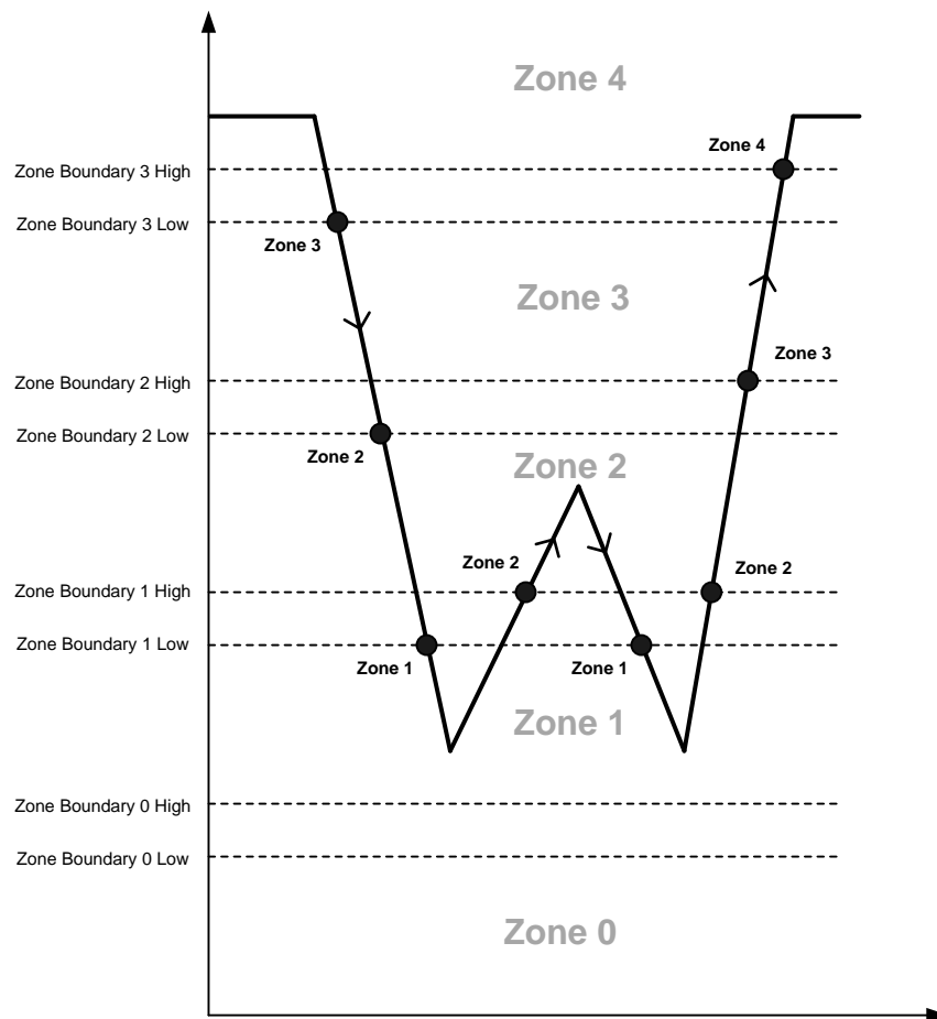
Figure 7. ALS Zone Boundary + Hysteresis
