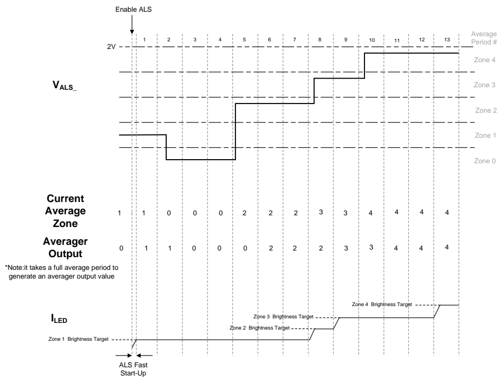
Figure 13. ALS Up-Only Control
