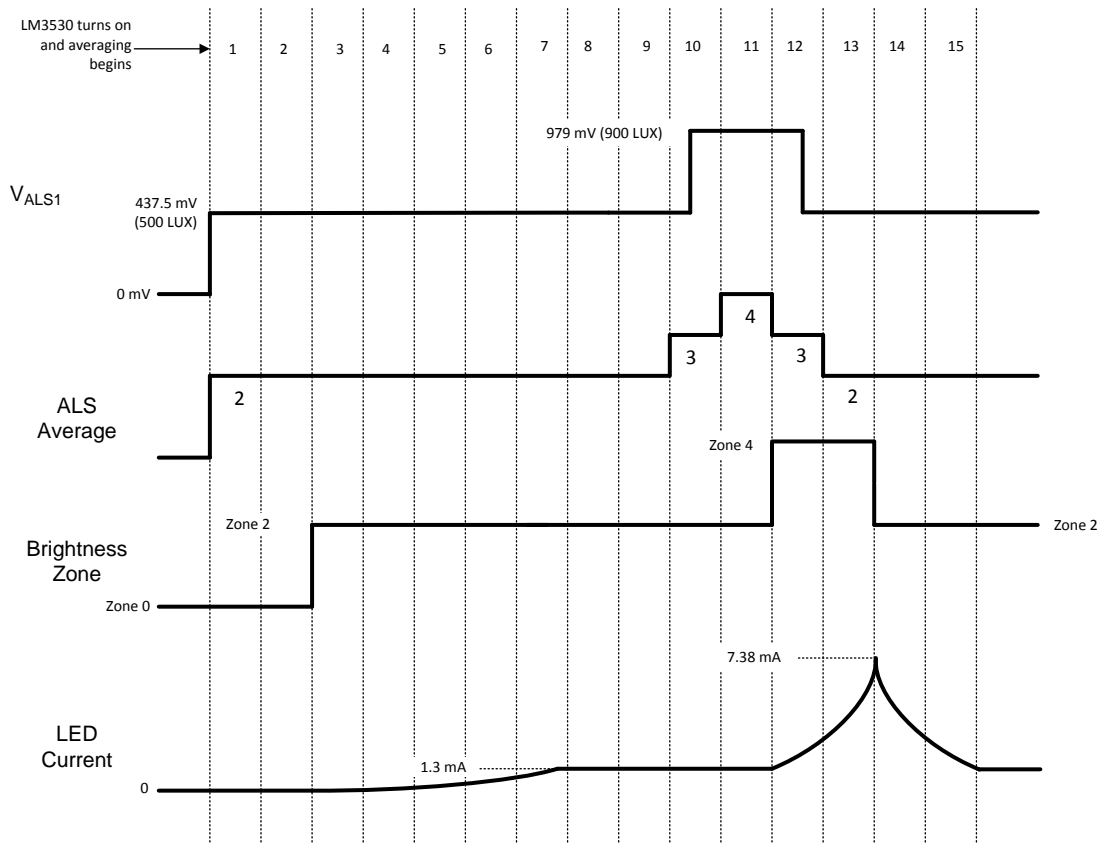
Figure 44. ALS Averaging Example
