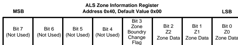
Figure 51. ALS Zone Information Register
