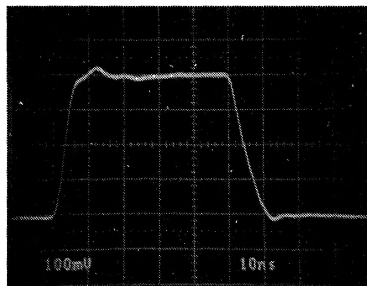
-- GND TL/H/9178-15
