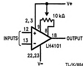
Offset Null
