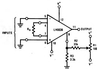
FIGURE 4. V OG Adjustment Circuit
