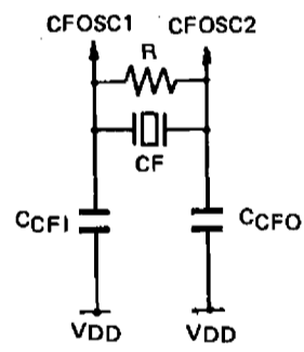
Fig. 13 CF oscillation
