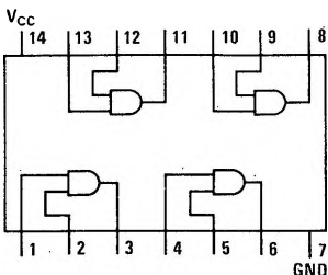
DM74H08
