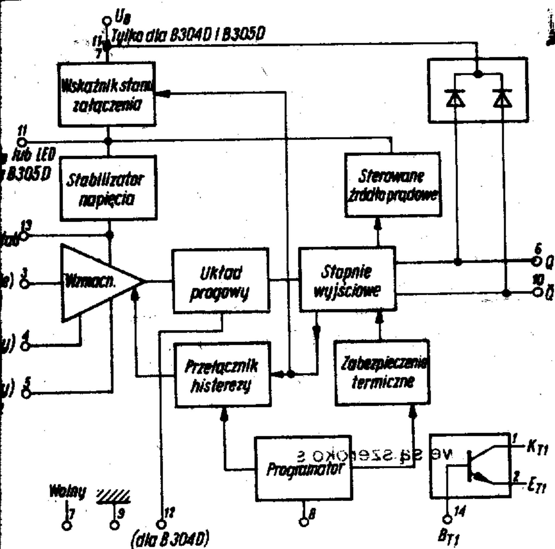
rys. 4. Schemat monolitycznych układów scalonych B303D, B304D i B305D (RFT).
