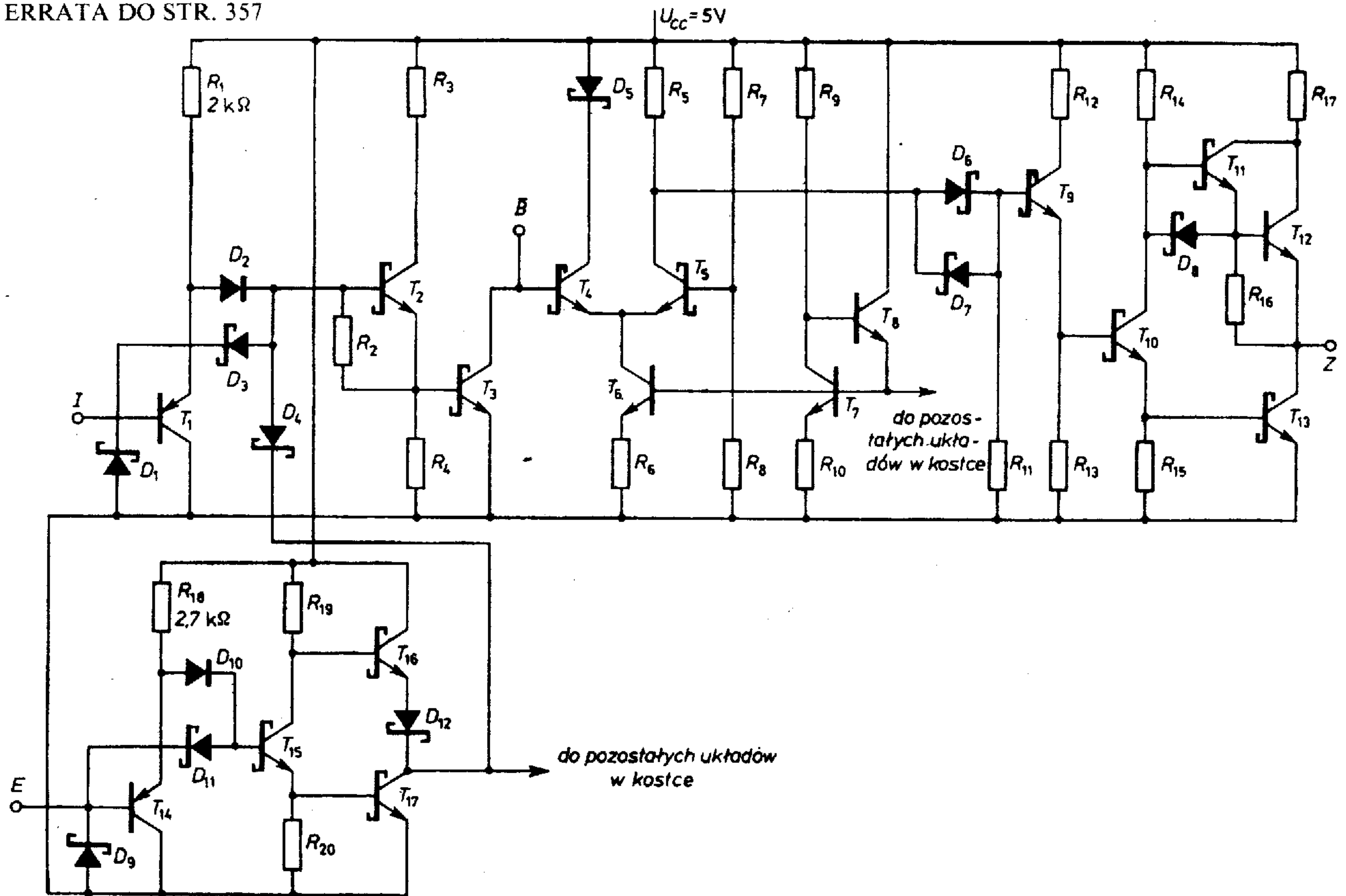
Rys. 6.36. Schemat układu Am26S10
